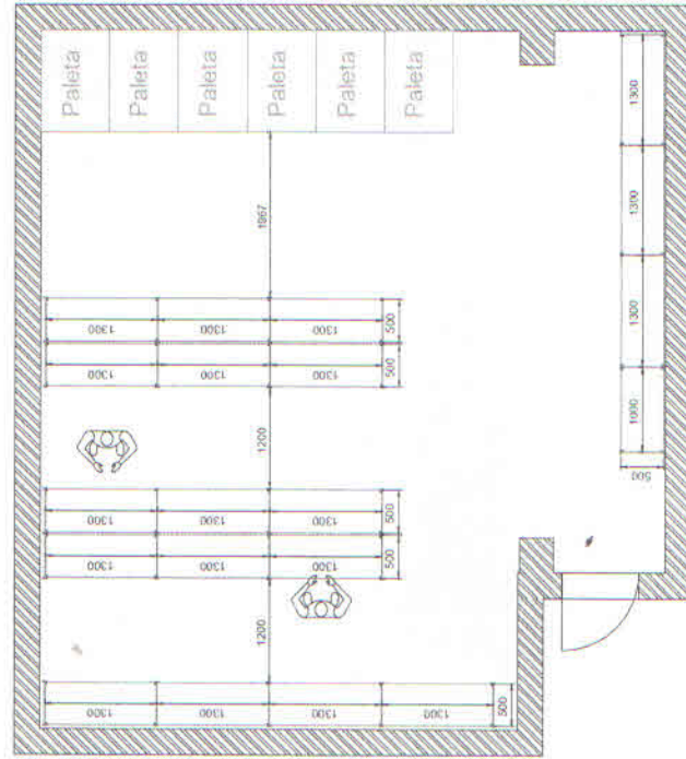
Pacienti suchý sklad - pôdorys
